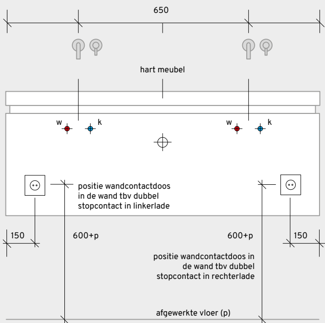
opstelling met enkele wastafel Saint Barth large of Saint Lucia large toepasbaar bij meubelbreedtes vanaf 1.200
