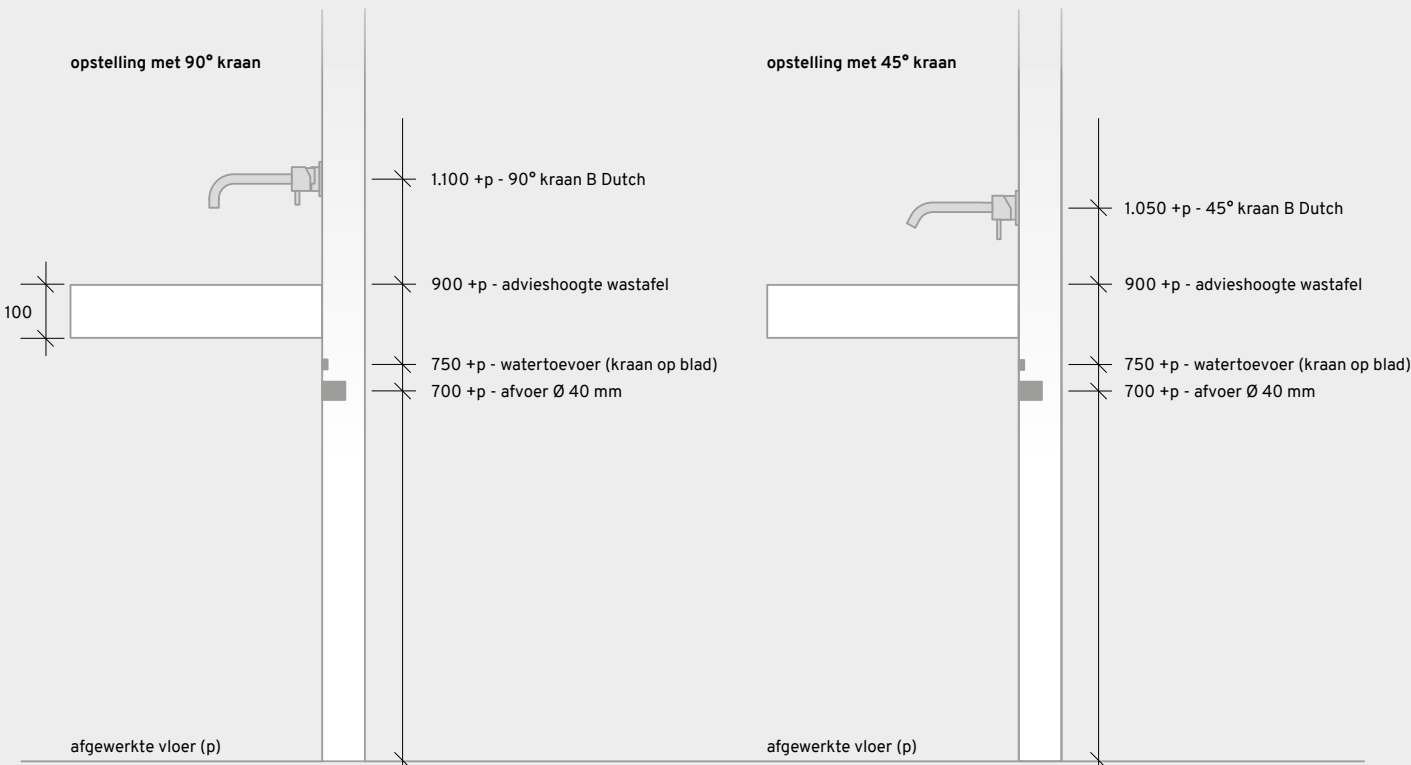
vooraanzicht opstelling met enkele wastafel large
