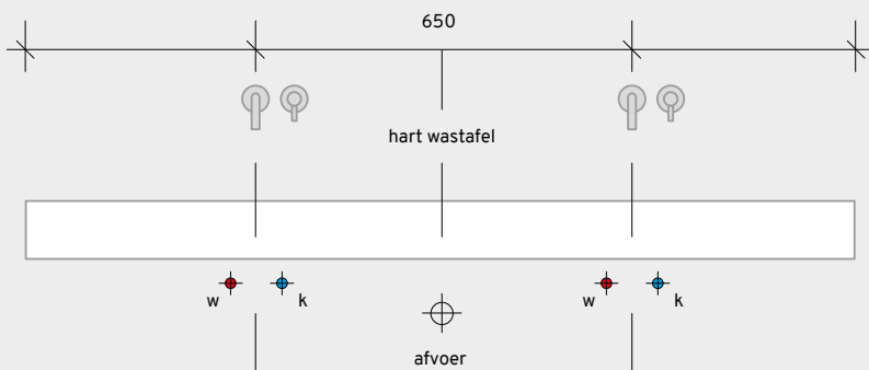
bovenaanzicht
