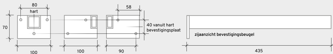
vooraanzicht bevestigingsbeugel breed
