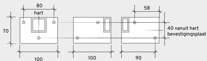
vooraanzicht bevestigingsbeugel breed
