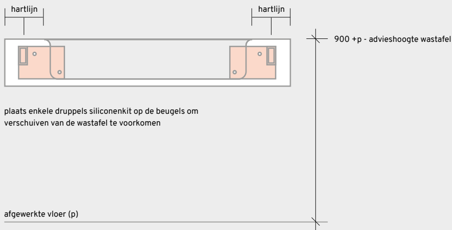
vooraanzicht
