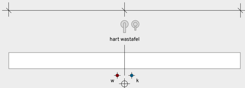
vooraanzicht opstelling met enkele wastafel small
