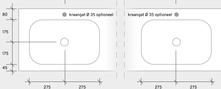
bovenaanzicht
