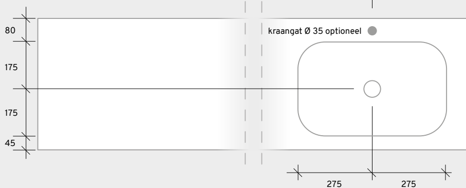
bovenaanzicht
