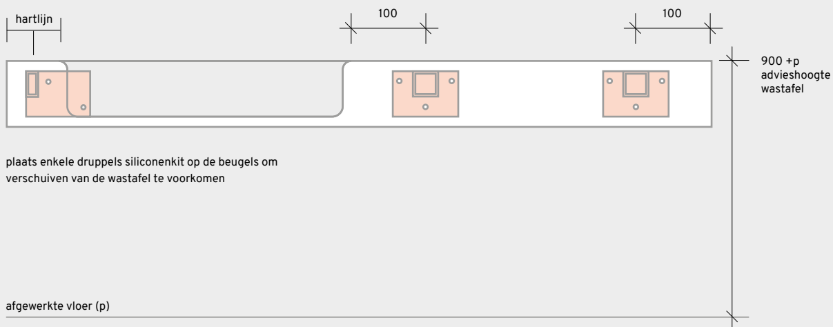
vooraanzicht
