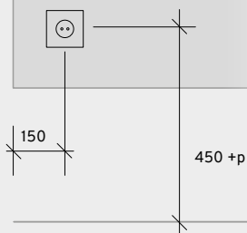
positie wandcontactdoos in de wand tbv dubbel stopcontact in linkerlade
