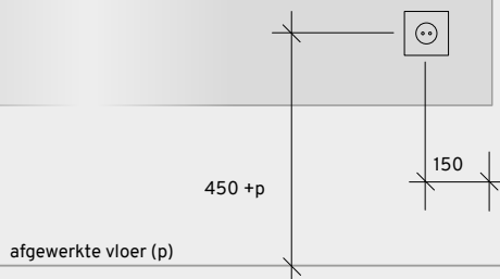
positie wandcontactdoos in de wand tbv dubbel stopcontact in rechterlade
